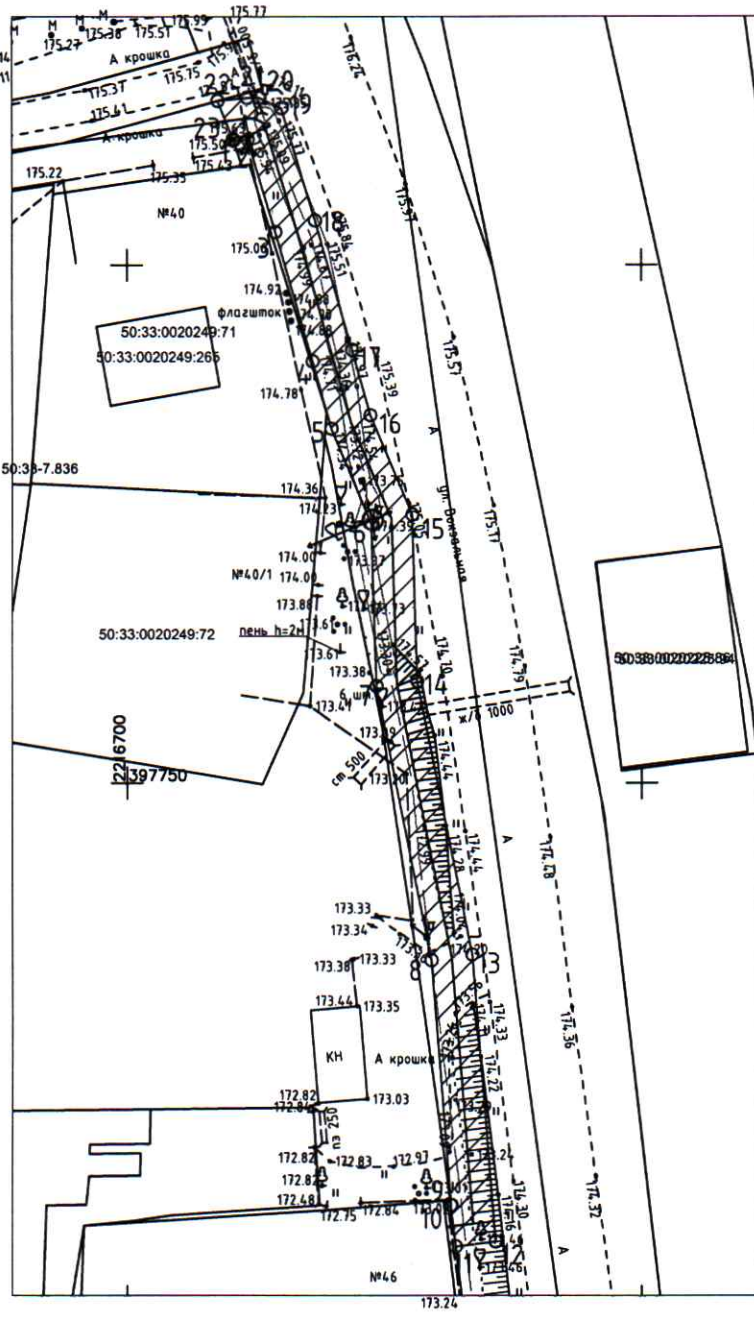
План масштаба 1:500
